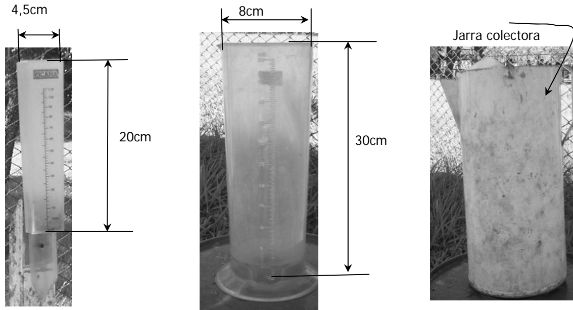
Figura n°7. Detalle del pluviómetro de cuña, probeta graduada y jarra colectora
